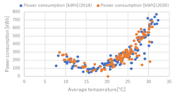
図3 2018年と2020年の平均気温と消費電力の関係
