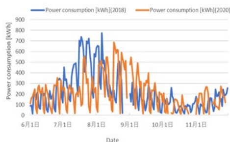
図1 2018年と2020年の電力比較
